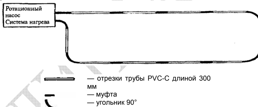
Рисунок 2 — Схема испытаний клеевых соединений труб и фитингов из PVC-C на стойкость к аварийной температуре T_{\text{авар}}
